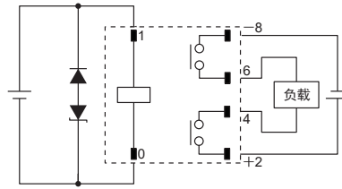
图4.反极性
