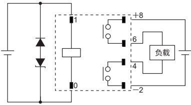
图3.正极性
