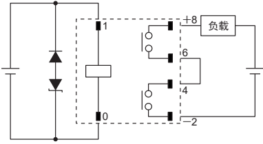
图1.正极性
